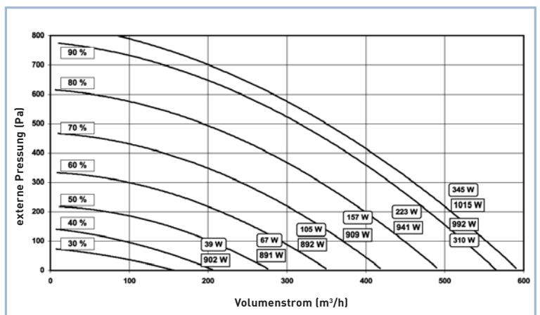
Diagramm 1: Kennlinie für Volumenstrom / externe Pressung / Leistungsaufnahme
