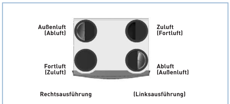
Bild 2: Geräteversionen
