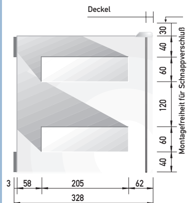
Ansicht Stirnseite
