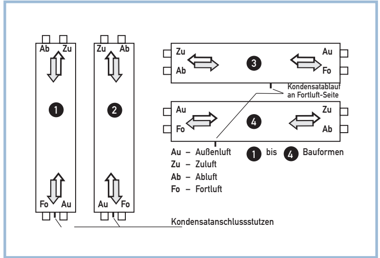
Bild 1: Bauformen
