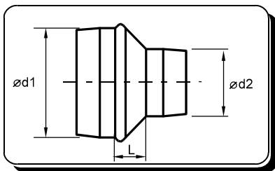
Reduzierung sym., kurze Ausführung aus verzinktem Stahlblech beidseitig mit Lippendichtung
