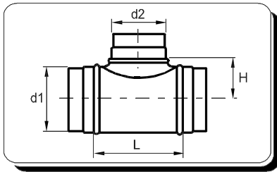
T-Stück aus verzinktem Stahlblech mit Lippendichtung
