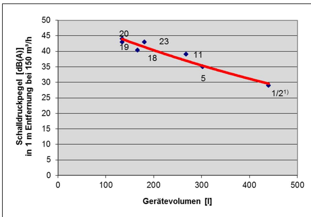
Bild 6: Abhängigkeit des Schalldruckpegels (1 m) vom Gerätevolumen (Ziffern im Diagramm = typische, marktgängige Geräte)
