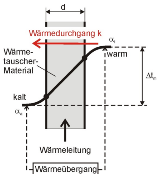
Bild 8: Wärmedurchgang
