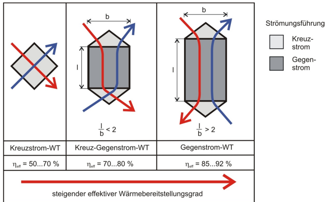
Bild 4: Strömungsformen in Wärmetauschern
