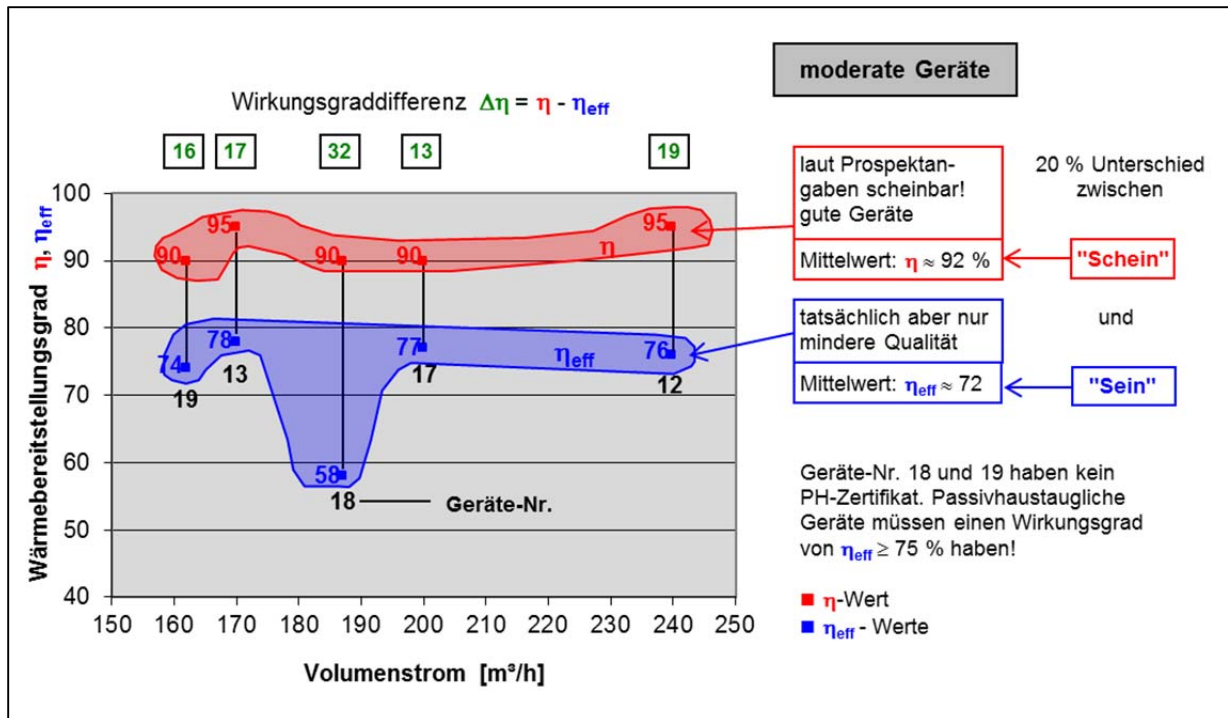
Bild 2: Bei weniger guten Wärmerückgewinnungsgeräten gemessene unterschiedliche Wärmebereitstellungsgrade:
