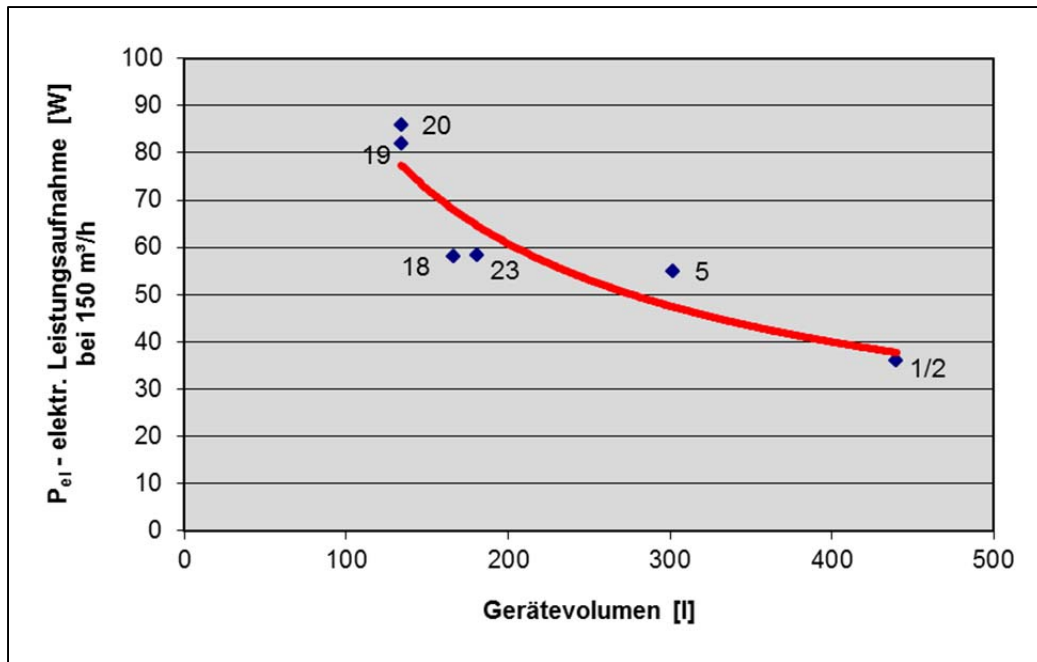
Bild 5: Abhängigkeit der Leistungsaufnahme vom Gerätevolumen (Ziffern im Diagramm = typische, marktgängige Geräte)
