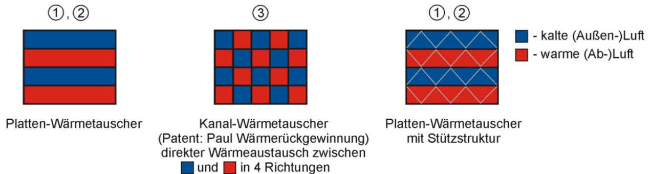
Bild 7: Plattenstruktur
