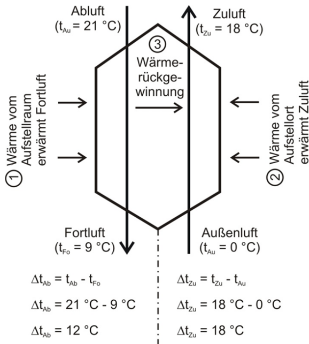
Bild 1: Einflussfaktoren auf die Lufterwärmung im WRG-Gerät
