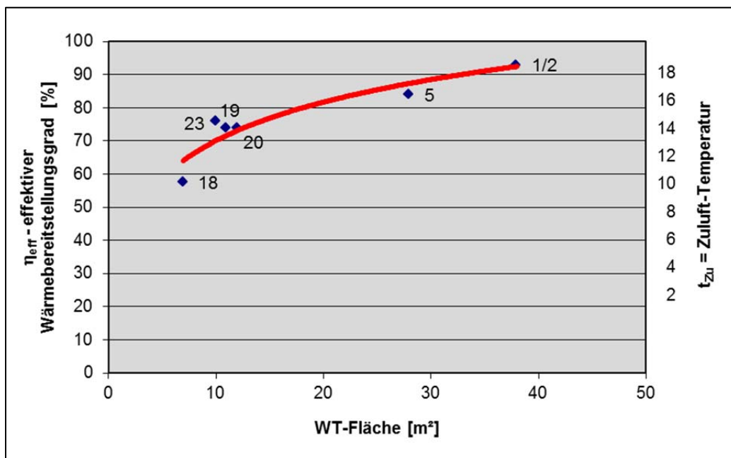
Bild 9: Abhängigkeit des Wärmebereitstellungsgrades von der WT-Fläche (Ziffern im Diagramm = typische, marktgängige Geräte)
