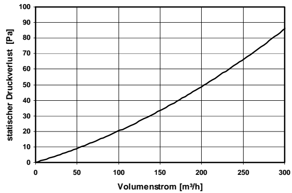
Aktivkohle-Filterkassette und Filterkassette F7
